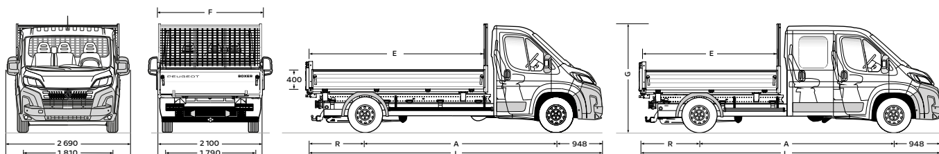
X250 Boxer Podwozie z wywrotką
