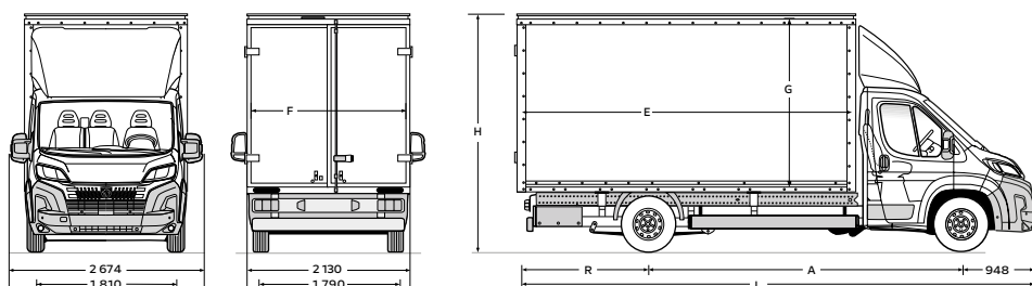
X250 Boxer Podwozie z kontenerem
