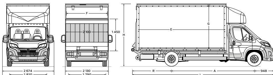
X250 Boxer Podwozie z kontenerem i windą hydrauliczną
